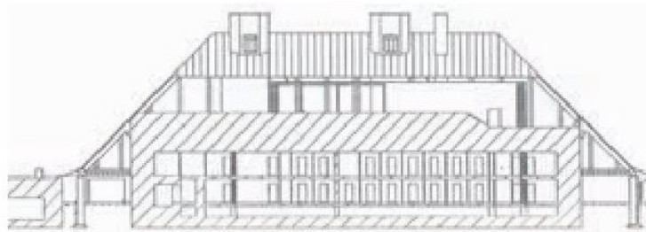
Doorsnede van de bunker van Seyss-Inquart aan de Van Brienenlaan. Collectie Ruud Pols, www.Bunkerarchie.nl .
